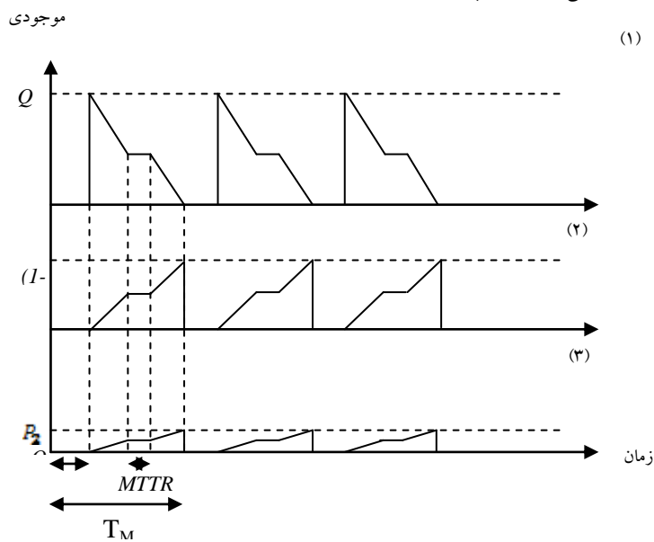
شکل ۱. نمودار موقعیت موجودی در جریان ساخت در حالت اعمال سیاست نت پیشگیرانه به ترتیب برای (۱) قطعات خام، (۲) محصولات سالم و (۳) ضایعات
