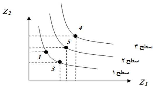
شکل ۱: مثالی از رده‌بندی نقاط غیر مغلوب به صورتی
