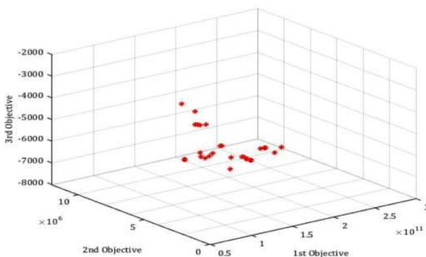
شکل ۵- شکل جبهه جواب الگوریتم MOPSO
